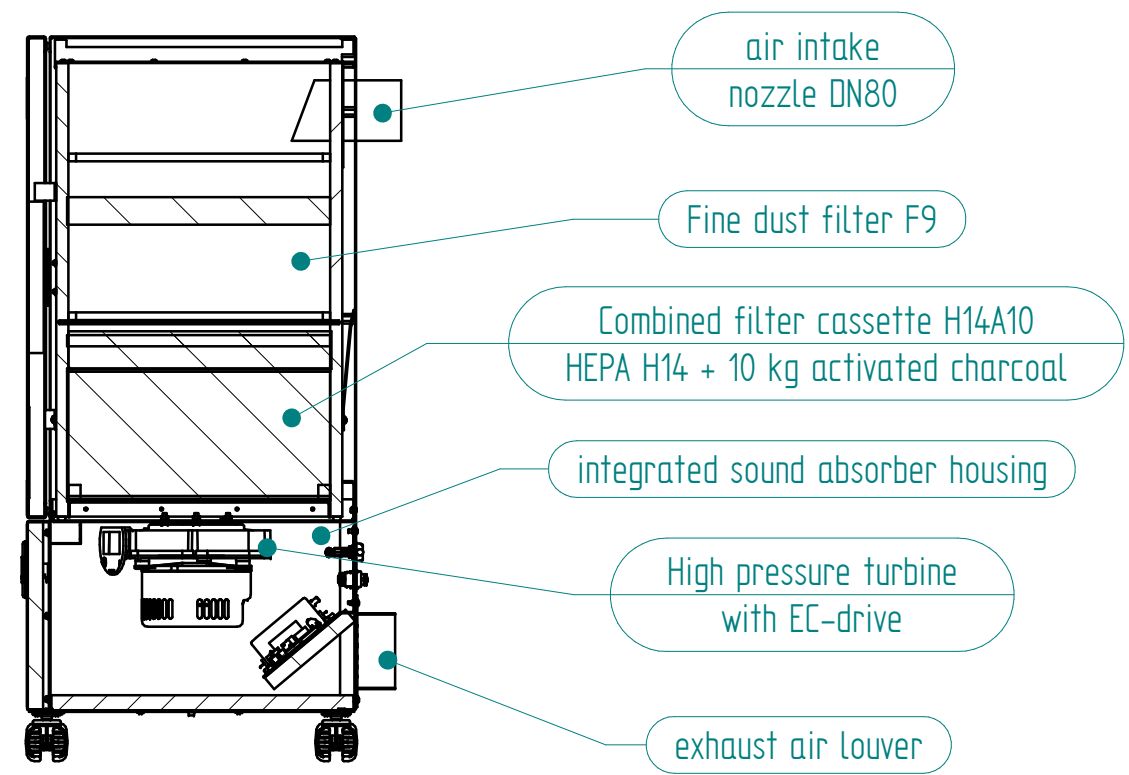
cutawayt C-C
